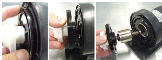
Läufer am Impeller packen und vorsichtig komplett rausziehen. Bauteile auf Verkalkungen überprüfen.
